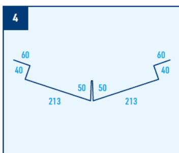
Úžlabí s drážkou, r.š. 725 mm
