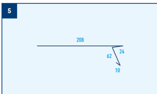
Lišta okapní, r.š. 304 mm
