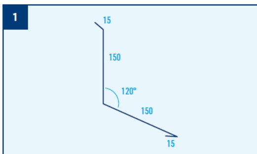
Lemování zdiva, r.š. 330 mm
