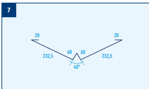
Lišta úžlabí se stojatou drážkou, r.š. 625 mm
