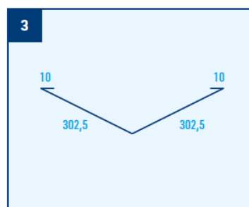
Úžlabí, r.š. 625 mm
