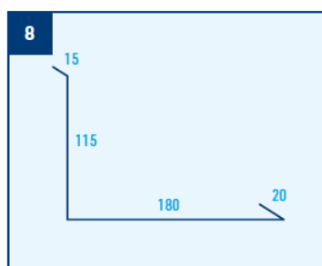
Lišta boční plochá, r.š. 330 mm
