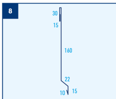
Lišta závětrná plochá nízká, r.š. 252 mm
