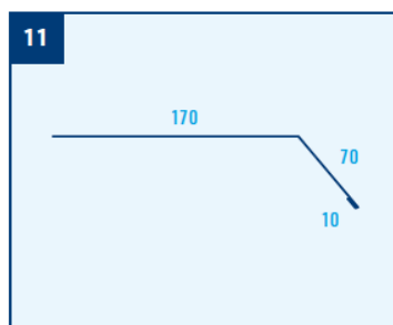
okapové lemování, r.š. 250 mm
