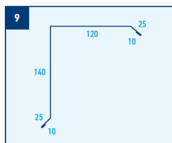
Lišta závětrná horní, r.š. 330 mm
