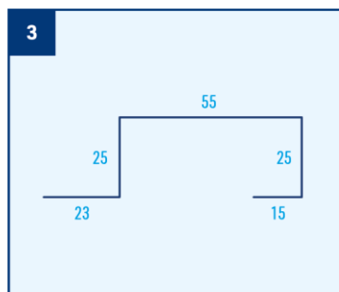
Lišta hřebenová větrací, r.š. 143 mm
