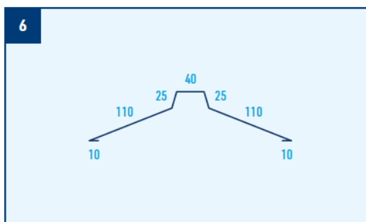
Hřebenáč (hladký), r.š. 330 mm
