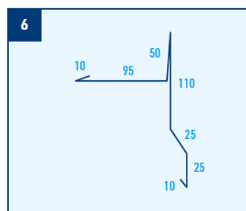
Lišta závětrná spodní, r.š. 333 mm
