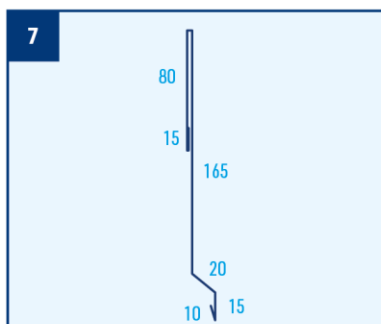
Lišta závětrná plochá, r.š. 305 mm
