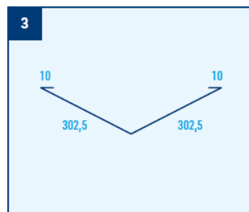
Úžlabí, r.š. 625 mm
