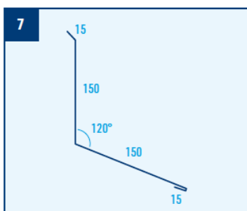
Lemování zdiva, r.š. 330 mm
