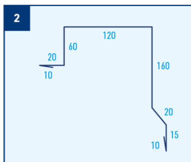
Lišta závětrná horní, r.š. 415 mm
