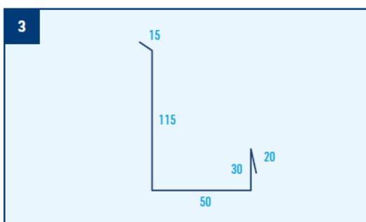
Lišta boční (plochá), r.š. 230 mm
