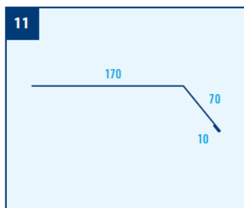
okapové lemování, r.š. 250 mm
