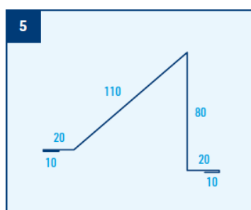
Sněhový zachytávač, r.š. 250 mm
