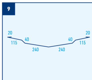
Lišta úžlabí, r.š. 830 mm
