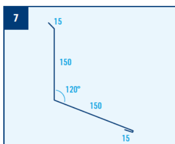
Lemování zdiva, r.š. 330 mm
