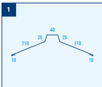
Hřebenáč hladký, r.š. 330 mm
