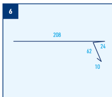
Lišta okapní, r.š. 304 mm
