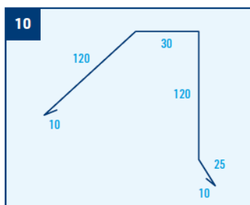
Pultové ukončení, r.š. 315 mm
