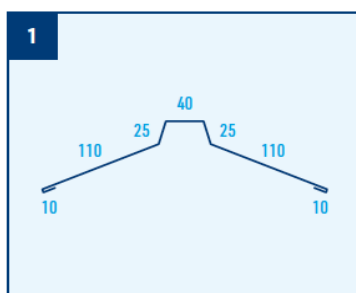
Hřebenáč hladký, r.š. 330 mm
