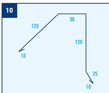
Pulťové ukončení, r.š. 315 mm
