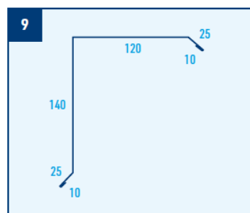
Lišta závětrná horní, r.š. 330 mm
