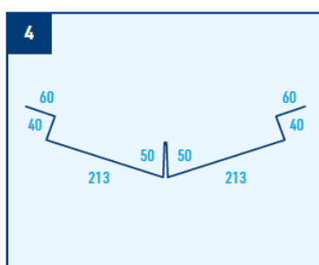
Úžlabí s drážkou, r.š. 725 mm
