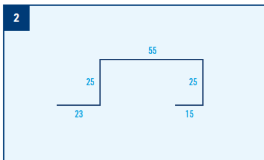
Lišta hřebenová (větrací), r.š. 143 mm
