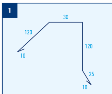
Pultové ukončení, r.š. 315 mm
