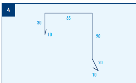
Lišta závětrná, r.š. 225 mm
