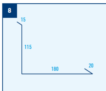
Lišta boční plochá, r.š. 330 mm
