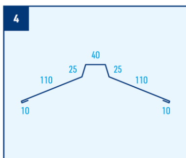
Hřebenáč hladký, r.š. 420 mm
