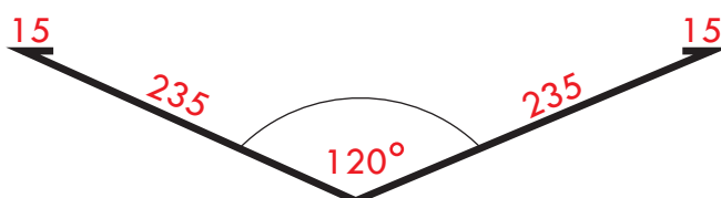
Lišta úžlabí r.š. 500 mm č. 7a
