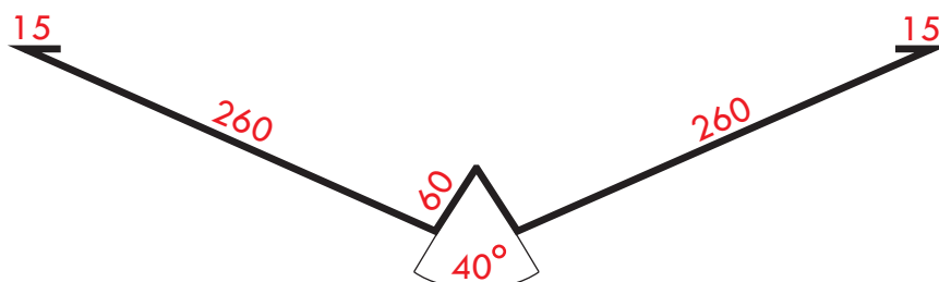
Lišta úžlabí se stojatou drážkou r.š. 670 mm č. 6b
