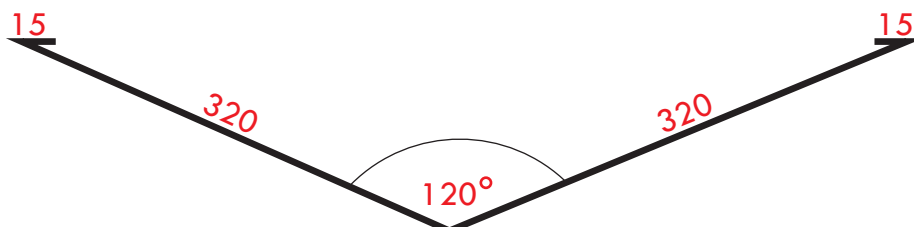
Lišta úžlabí r.š. 670 mm č. 7b
