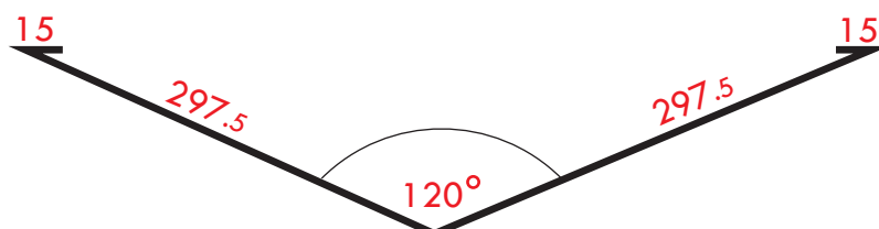
Lišta úžlabí r.š. 625 mm č. 7c
