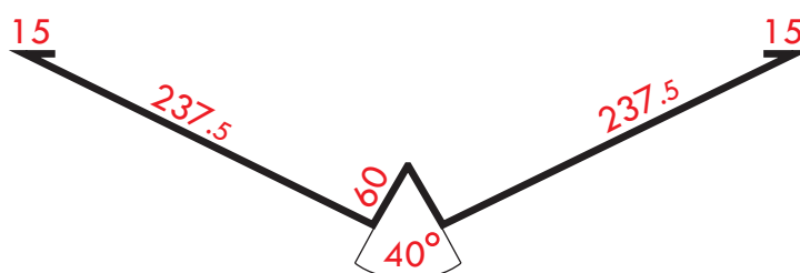
Lišta úžlabí se stojatou drážkou r.š. 625 mm č. 6c
