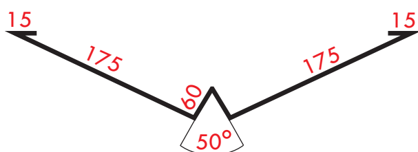
Lišta úžlabí se stojatou drážkou r.š. 500 mm č. 6a
